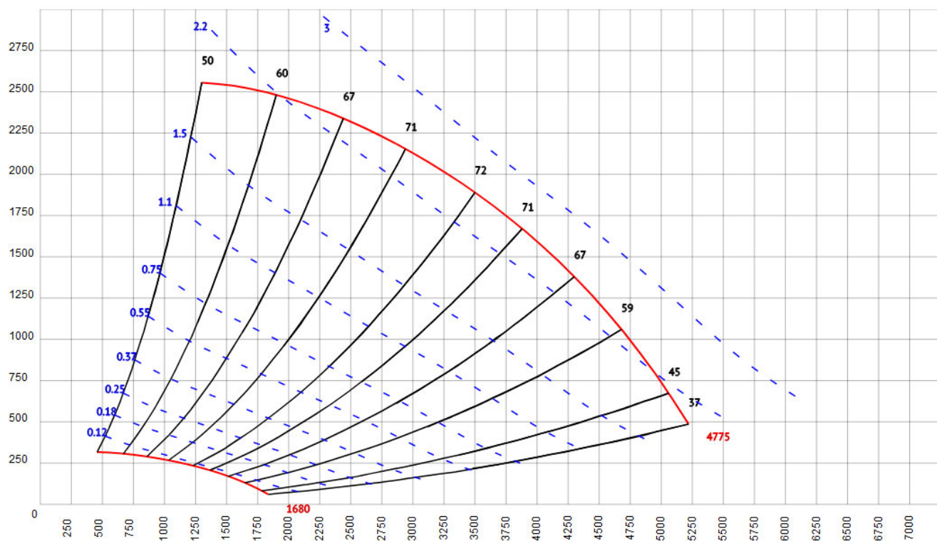
Рис.8. КЦ-280
