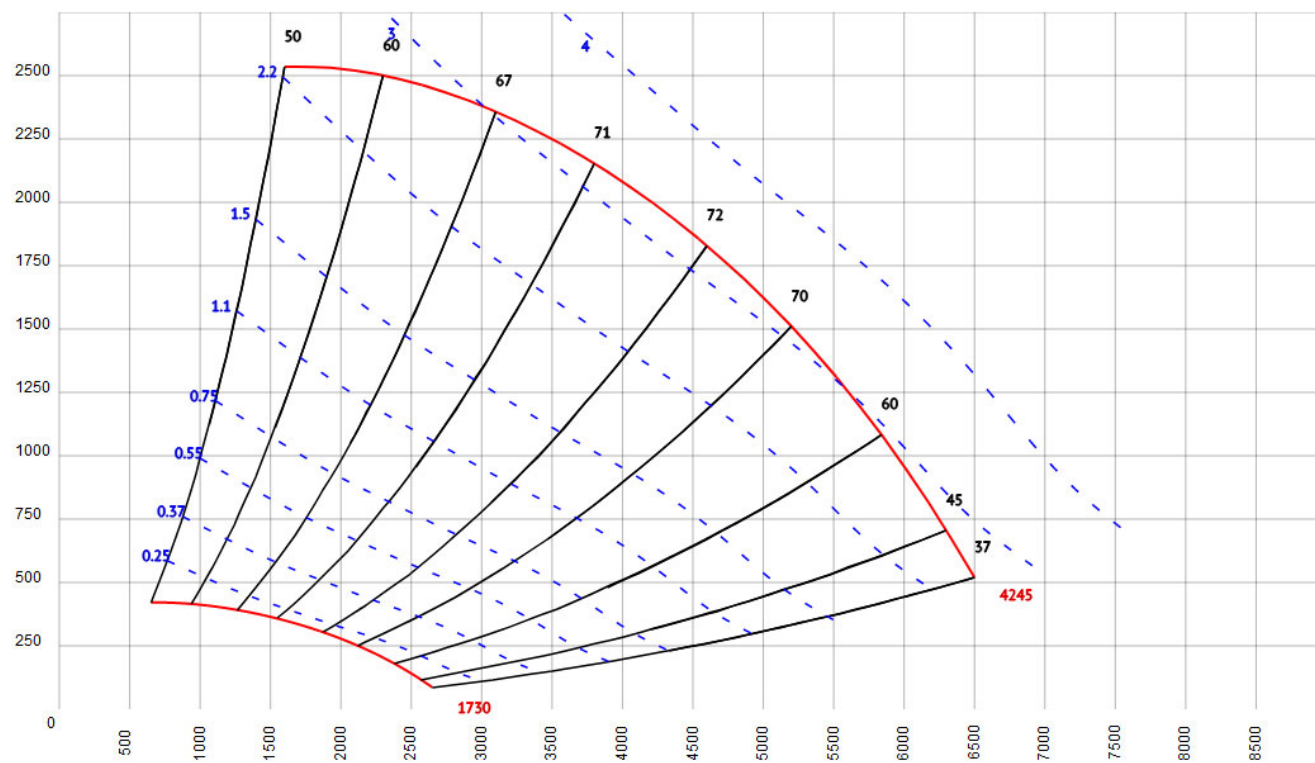
Рис.9. КЦ-310
