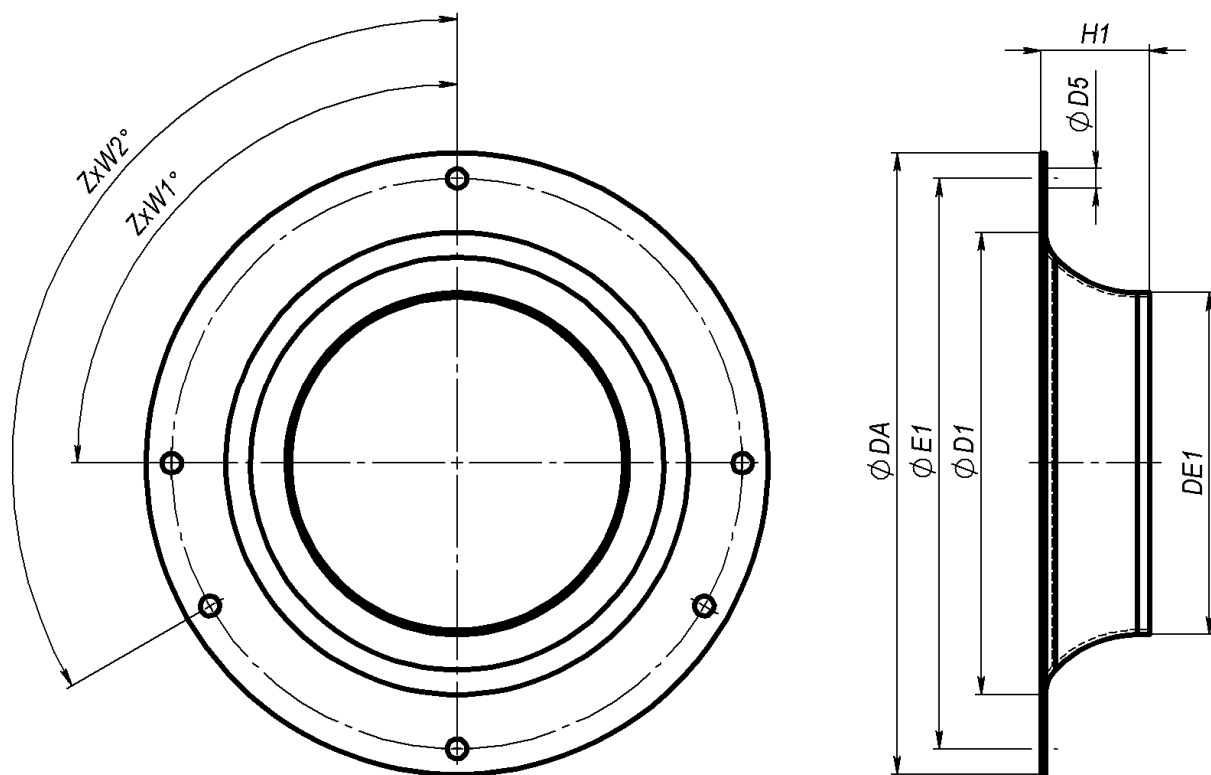
Рис. 1.2. Геометрические характеристики конфузора
