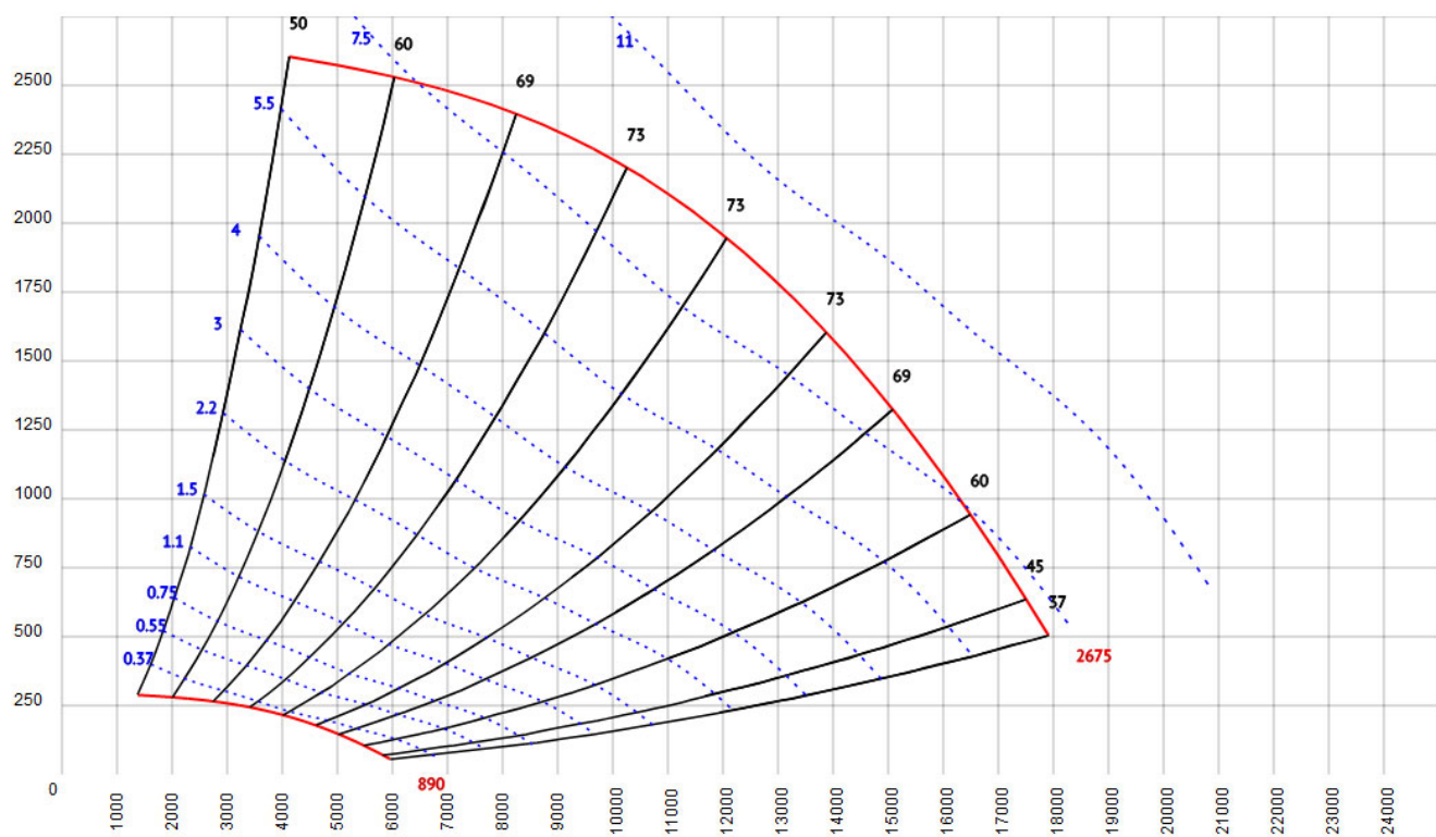
Рис.13. КИ-500
