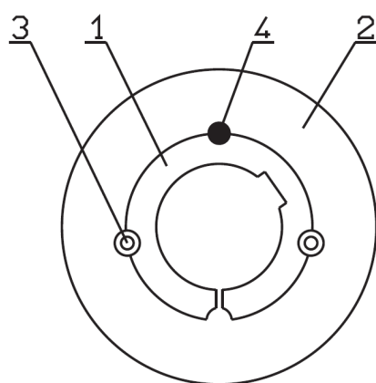
Рис.22. Монтаж КЦ
