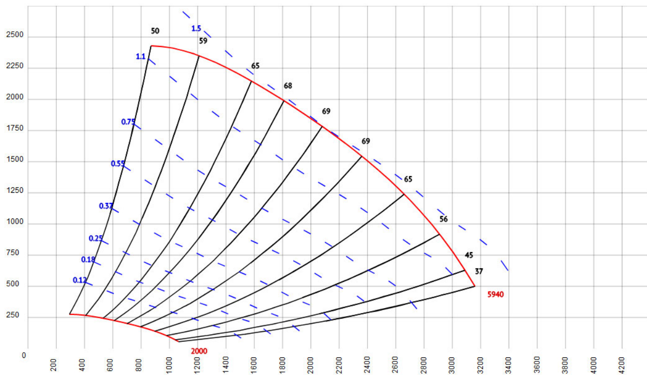
Рис.6. КЦ-220
