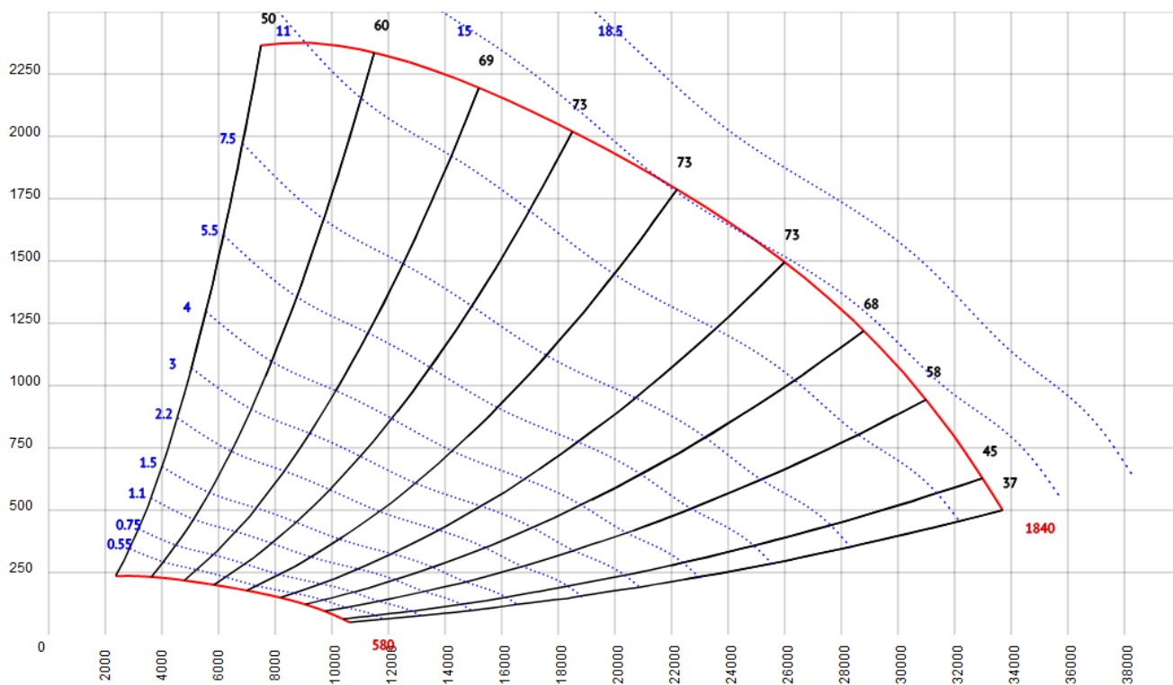
Рис.16. КЦ-710
