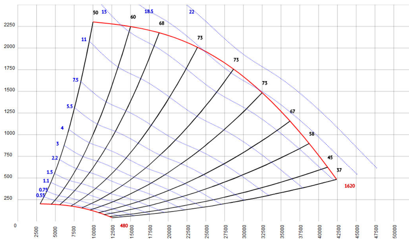
Рис.17. КЦ-800
